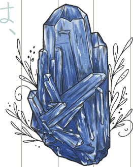
\text{Al}_2\text{SiO}_5
